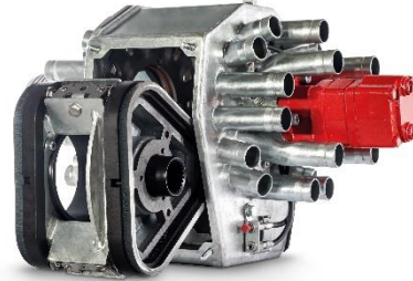
Bild 4: Durch verbaute Exzenternachsteller ist der Exaktverteiler ExaCut ECQ schneidkräftig und widerstandsfähig.
